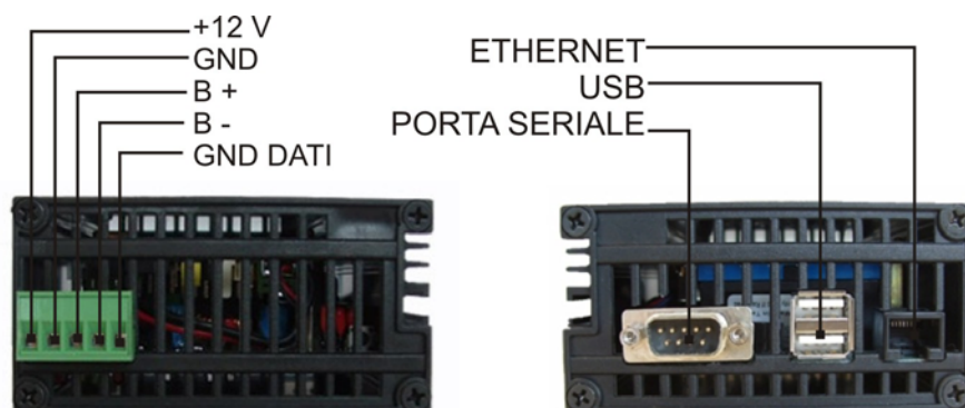
Fig.1: schema collegamenti
